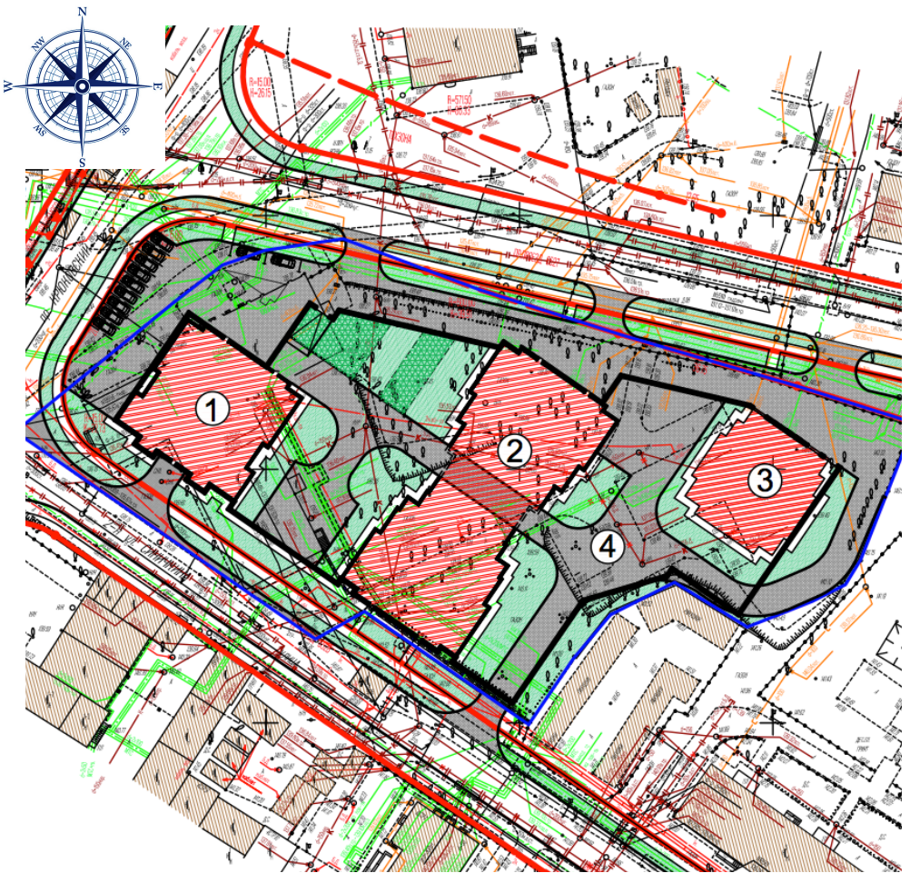
Схема генерального плана
